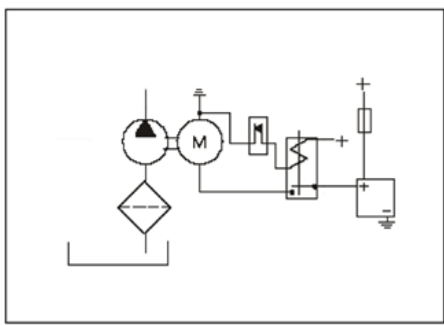
Рисунок 1.2 Схема подключения
